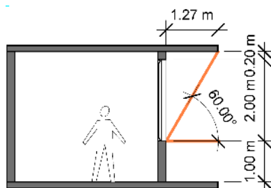
شکل ۳: عمق سایبان
