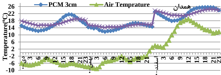
شکل ۸. مقایسه‌ی دمای داخلی سقف با ماده تغییر فاز دهنده و سقف مرجع در فصول مختلف برای همدان و بوشهر
