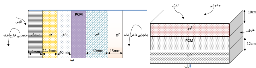
شکل ۱. ساختار سقف (الف) و دیوار (ب)
