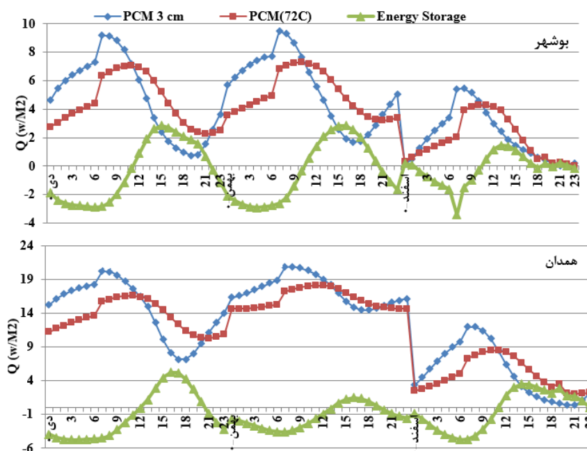
شکل ۱۰. مقایسه‌ی شار حرارتی آنی اتلافی در زمستان در بوشهر و همدان
