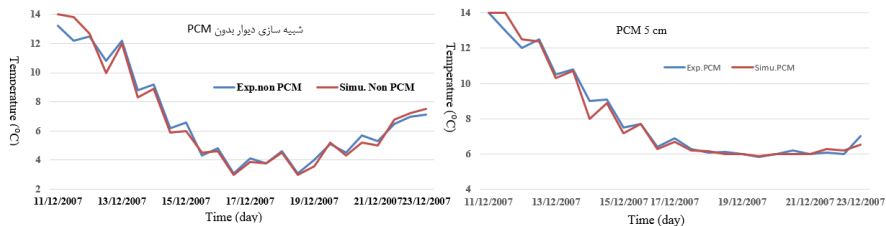
شکل ۶. مقایسه‌ی نتایج تجربی (پسوپاتی، ۲۰۰۸) و شبهه‌سازی دمای داخلی دیوار
