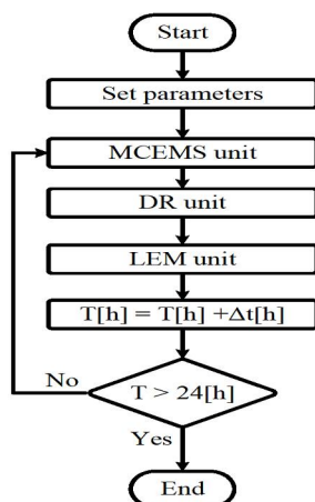
شکل (۱) روندنمای الگوریتم MCEMS_LEM
