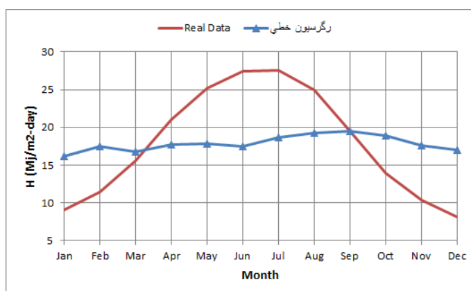
نمودار ۳. مقایسه مقادیر تجربی و برآورد شده تابش خورشیدی با استفاده از روش رگرسیون خطی (رابطه ۱۸)
