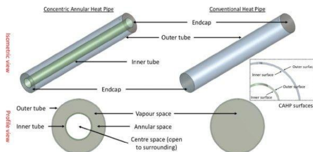
شکل ۷: مقایسه‌ای بین عملکرد لوله حرارتی متعارف و لوله حرارتی حلقوی هم‌مرکز که طراحی دایره‌ای آن باعث بهبود توزیع شار حرارتی و بازده انتقال حرارت می‌شود (چُهوکر و همکاران ۶۴ ، ۱۴۰۳)
