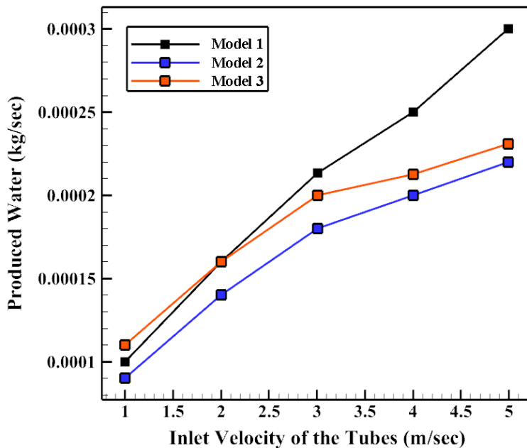
شکل ۱۰. آب تولیدی بر حسب سرعت‌های ورودی لوله برای مدل‌های مختلف
