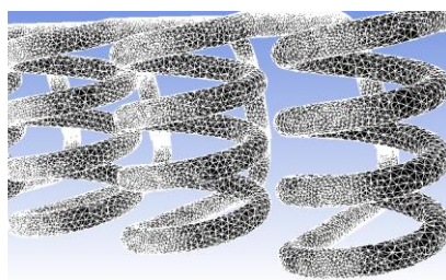
شکل ۲. الف) شماتیک مبدل حرارتی مورد استفاده برای صحت‌سنجی (ب) شبکه‌بندی ایجاد شده در هندسه مورد بررسی
