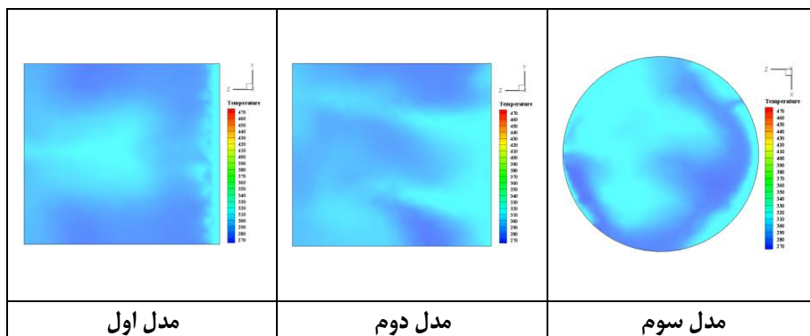
شکل ۱۲. کانتور دما در خروجی پوسته برای مدل‌های مختلف در V=3 \text{ m/sec}
