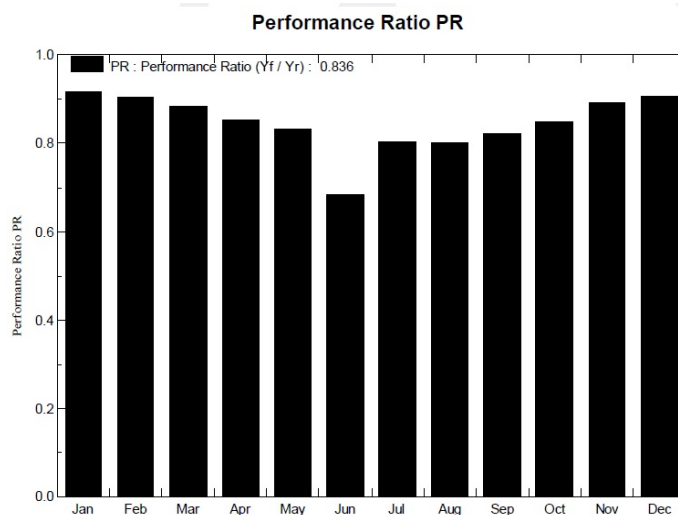
شکل ۳) میانگین ضریب عملکرد (PR)
