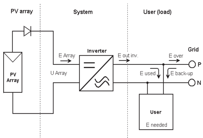
شکل (۱) سیستم فتوولتائیک متصل به شبکه
