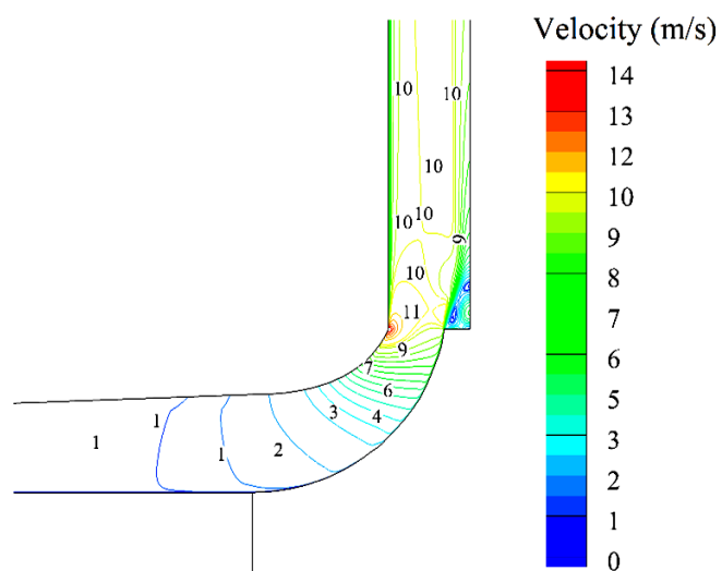
شکل ۷. کانتور سرعت برای شرایط آب و هوایی شهر اهواز
