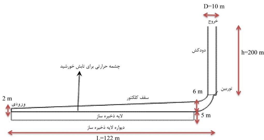
شکل ۲. مشخصات هندسی نیروگاه دودکش خورشیدی مورد مطالعه و مانزائارس (اسپانیا)
