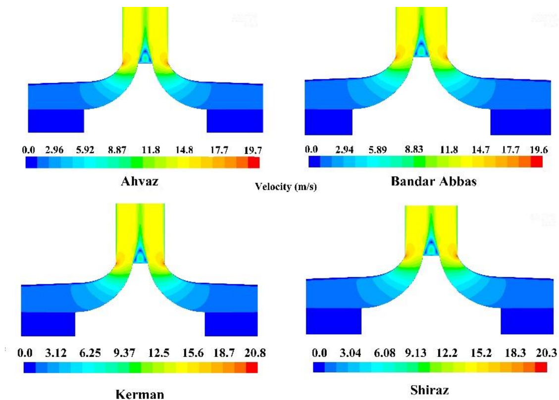
شکل ۸. کانتور سرعت برای شهرهای مختلف
