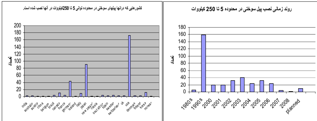
شکل (۱۱ و ۱۰): روند زمانی و محل نصب پیل‌های سوختی نصب شده در محدوده توانی ۵ تا ۲۵۰ کیلووات
