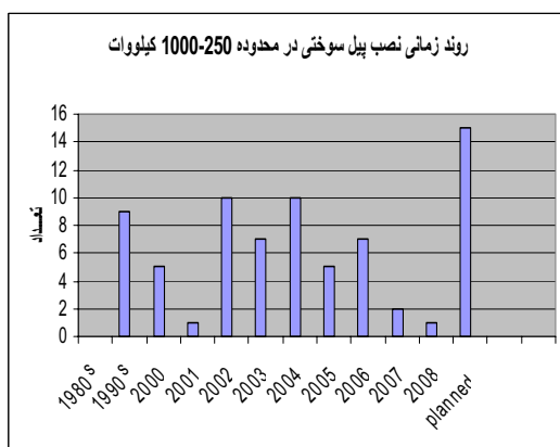
شکل (۷و۶): روند زمانی و محل نصب پیل‌های سوختی نصب شده در محدوده توانی ۲۵۰ تا ۱۰۰۰ کیلووات
