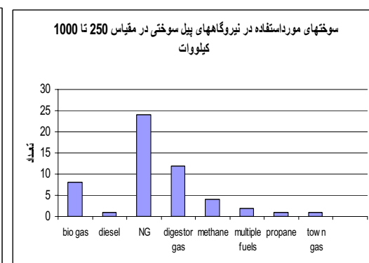
شکل (۹و۸): سوخت‌های مورد استفاده و انواع پیل‌های سوختی نصب شده در محدوده توانی ۲۵۰ تا ۱۰۰۰ کیلووات
