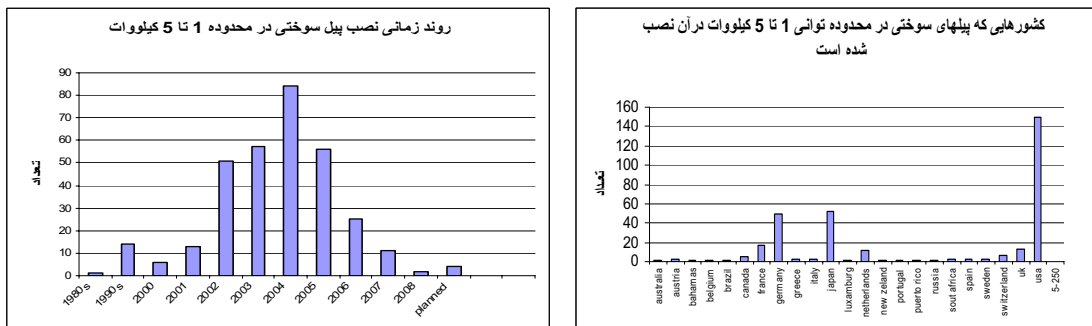
شکل (۱۴ و ۱۵): روند زمانی و محل نصب پیل‌های سوختی نصب شده در محدوده توانی ۱ تا ۵ کیلووات
