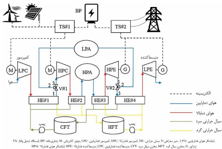
شکل ۸. نمای شماتیک و جریان انرژی سیستم ذخیره‌سازی انرژی هوای فشرده زیرآبی چندسطحی در دو سطح [۵۵]
