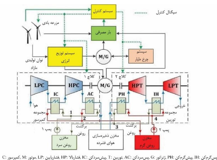
شکل ۷. طرح شماتیک سیستم ترکیبی سیستم ذخیره‌سازی انرژی چرخ طیار و ذخیره‌سازی انرژی هوای فشرده بی‌دررو [۶۸]
