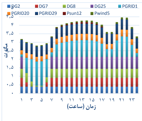
شکل ۵-۲. نمودار میانگین مشارکت تأمین بار الکتریکی واحدها با منابع CHP و بدون برنامه پاسخ‌گویی بار
