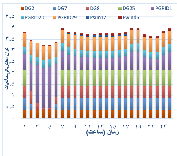
شکل ۵-۳. نمودار میانگین مشارکت تأمین بار الکتریکی واحدها بدون منابع CHP و با برنامه پاسخ‌گویی بار
