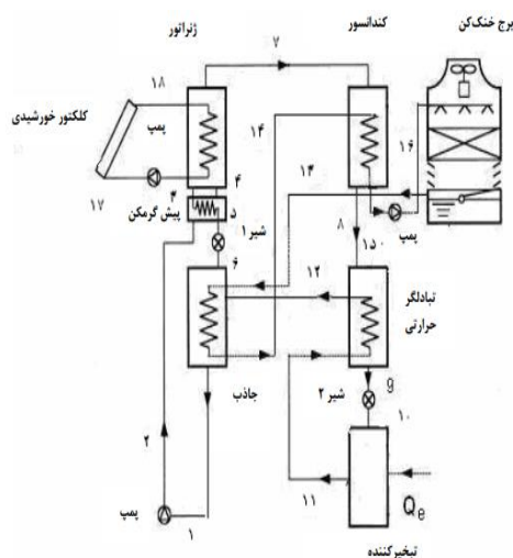
شکل ۱ یک سیکل جذبی خورشیدی
