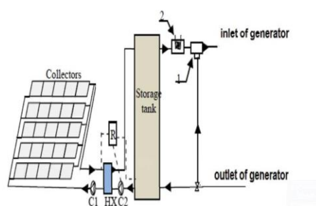
شکل ۱ شماتیک سیستم خورشیدی در چیلر جذبی خورشیدی
