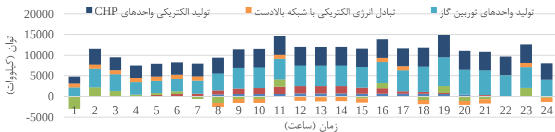
شکل ۱۱: تولید الکتریکی منابع مختلف در شبکه ۱۸ شین برای ۲۴ ساعت در حالت سوم از دسته اول
