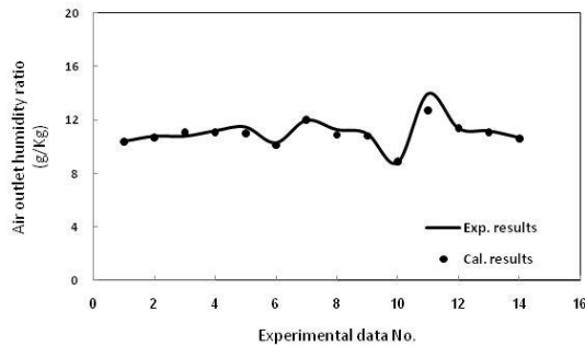
شکل ۵: مقایسه نتایج تحلیلی و تجربی (نسبت رطوبت هوا در خروجی رطوبت‌زدا)
