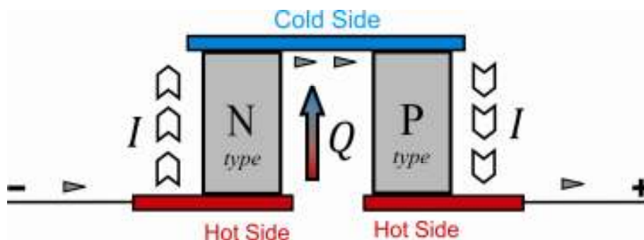
شکل ۲) نحوه عملکرد یک زوج ترموالکتریک شامل قرص‌های ترموالکتریک نوع N و P
