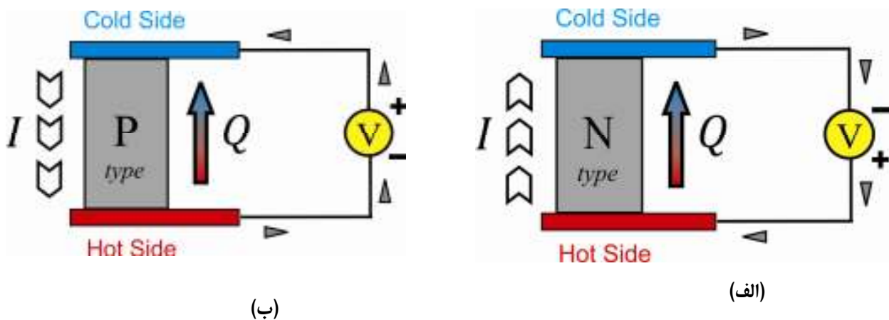
شکل ۱) نحوه عملکرد قرص‌های ترموالکتریک نوع P و N
