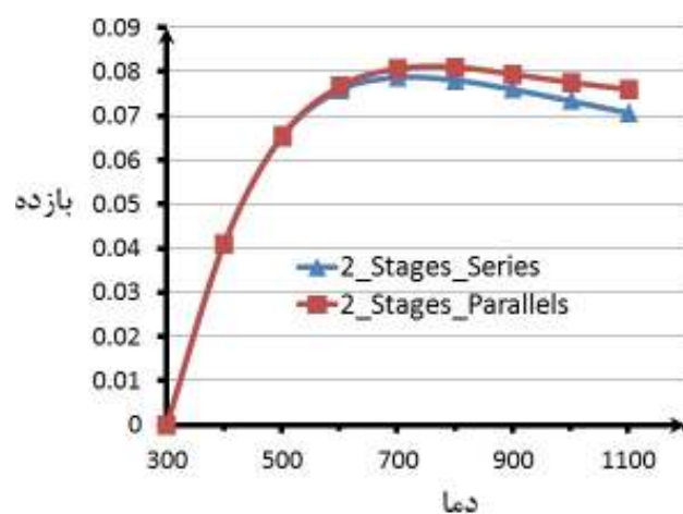
شکل ۸) نمودار بازده بر حسب دمای سطح گرم در سیستم‌های ژنراتور ترموالکتریک دومرحله‌ای سری و موازی ( T_c = 300\text{ K} )
