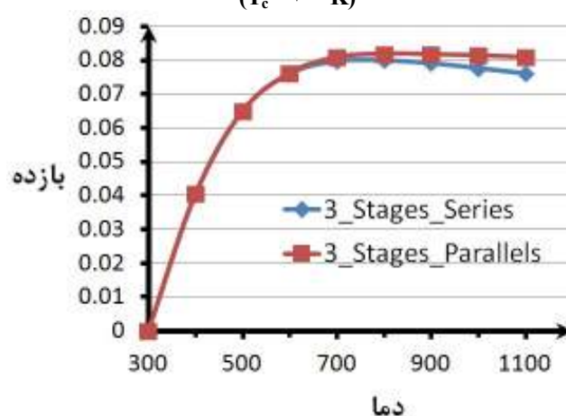
شکل ۹) نمودار بازده بر حسب دمای سطح گرم در سیستم‌های ژنراتور ترموالکتریک سه‌مرحله‌ای سری و موازی ( T_c = 300\text{ K} )
