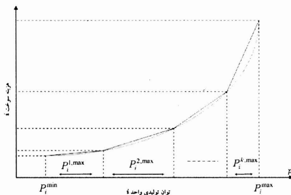
شکل (۲) تابع هزینه سوخت تکه ای خطی شده
