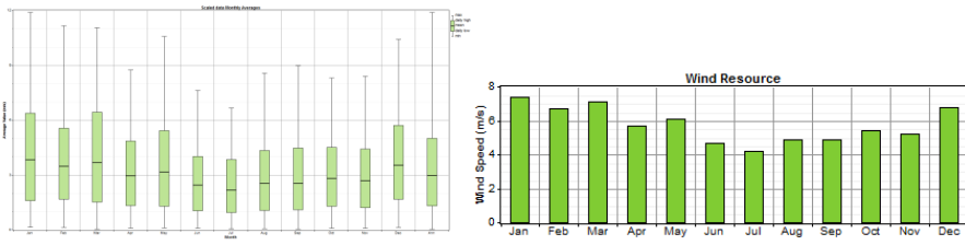
شکل ۷. میانگین سرعت وزش باد در ماه‌های مختلف سال
