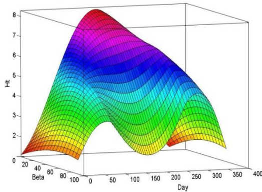
شکل ۱۲) روند تاثیر گذاری زاویه شیب بر میزان انرژی دریافتی به ازای زاویه آزیموت ثابت در روزهای مختلف سال.
