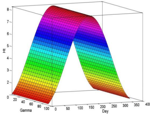
شکل ۱۱) روند تاثیر گذاری زاویه آزیموت بر میزان انرژی دریافتی به ازای زاویه شیب ثابت در روزهای مختلف
