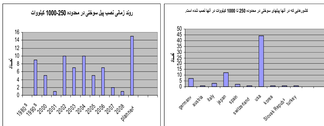
شکل (۷و۶): روند زمانی و محل نصب پیل‌های سوختی نصب شده در محدوده توانی ۲۵۰ تا ۱۰۰۰ کیلووات
