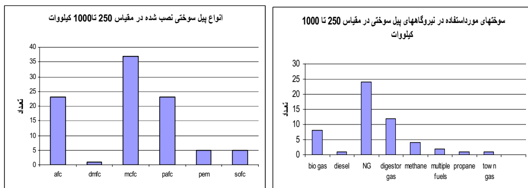
شکل (۹و۸): سوخت‌های مورد استفاده و انواع پیل‌های سوختی نصب شده در محدوده توانی ۲۵۰ تا ۱۰۰۰ کیلووات
