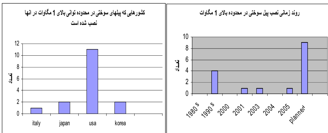
شکل (۵و۴): روند زمانی و محل نصب پیل‌های سوختی نصب شده در محدوده توانی بالای ۱ مگاوات
