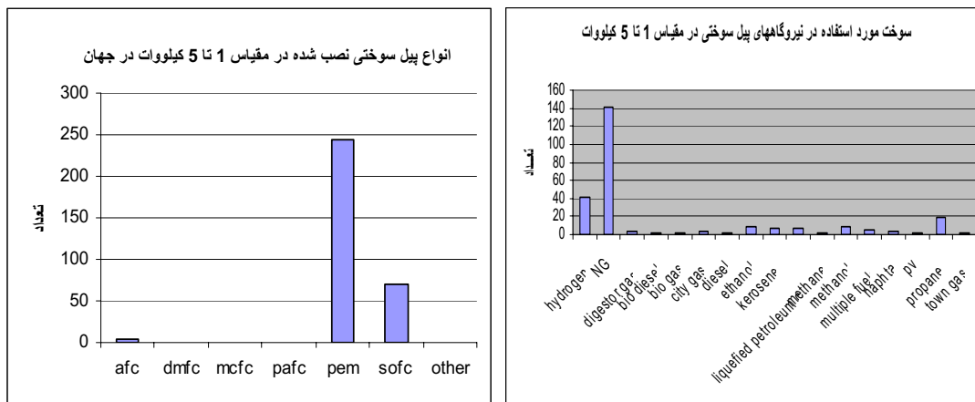
شکل (۱۷ و ۱۶): سوخت‌های مورد استفاده و انواع پیل‌های سوختی نصب شده در محدوده توانی ۱ تا ۵ کیلووات
