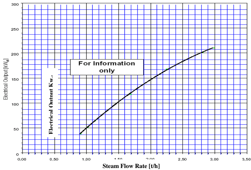
شکل ۶- تغییرات میزان برق تولیدی توسط ماشین بخار به ازای فشار ورودی 17/5 barg (حالت ارسال بخار اشباع به ماشین بخار)
