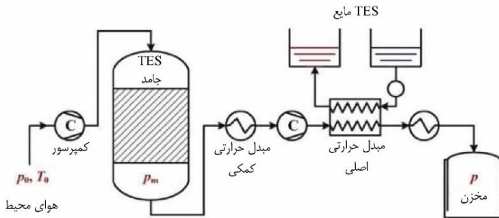
شکل ۴. نمای شماتیک سیستم ذخیره‌سازی انرژی هوای فشرده بی‌دررو ترکیبی در مرحله ذخیره‌سازی انرژی [۵۹]
