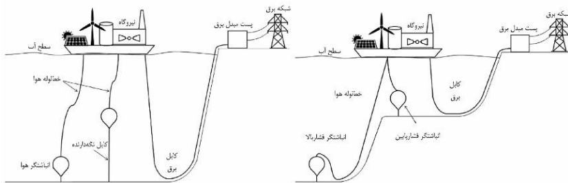
شکل ۹. نمونه‌هایی از طراحی‌های پیشنهادی برای سیستم ذخیره‌سازی انرژی هوای فشرده زیرآبی چندسطحی [۵۵]
