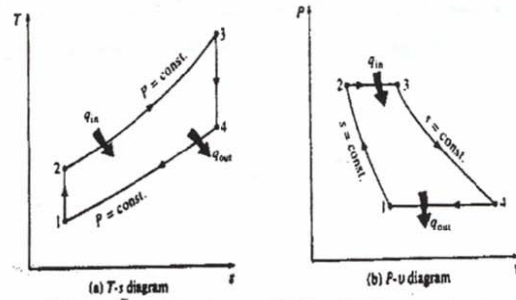
شکل ۲- نمودارهای T-S و P-V در سیکل ایده‌آل برایتون
