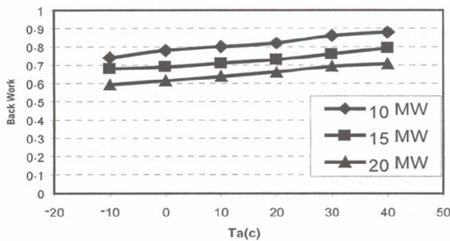
شکل ۱۱- اثر تغییر دمای محیط بر نسبت کار معکوس در توربین‌های گازی
