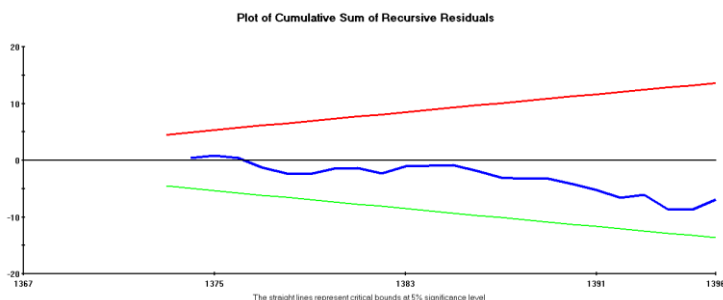
نمودار ۲. نتایج پایداری الگو با استفاده از آزمون CUSUM
