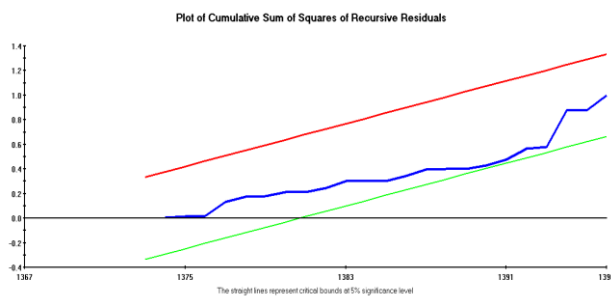
نمودار ۳. نتایج پایداری الگو با استفاده از آزمون CUSUMQ
