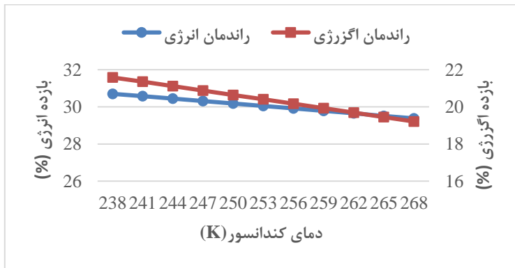
شکل ۴. تأثیر دمای کندانسور بر راندمان انرژی و راندمان انرژی ازگزرژی
