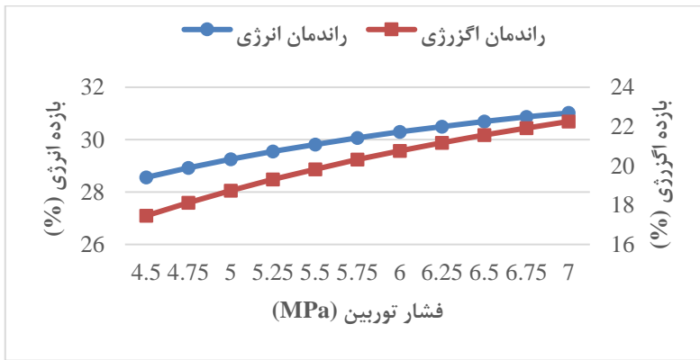
شکل ۳. تأثیر فشار توربین بر بازده انرژی و بازده انرژی ازگزرژی
