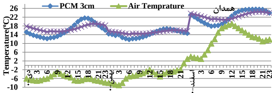
شکل ۸. مقایسه‌ی دمای داخلی سقف با ماده تغییر فاز دهنده و سقف مرجع در فصول مختلف برای همدان و بوشهر
