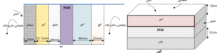
شکل ۱. ساختار سقف (الف) و دیوار (ب)
