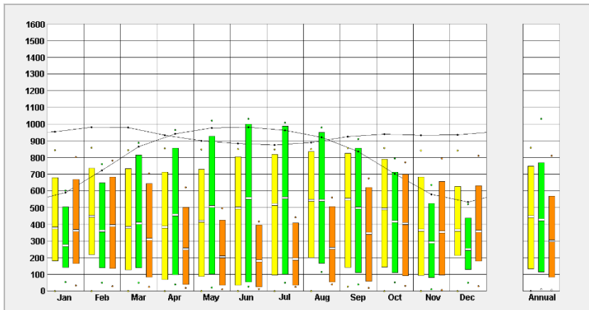
شکل ۴. میزان دریافت تابش خورشیدی (نگارندگان، از نرم‌افزار کلایمت کانسالتنت)
