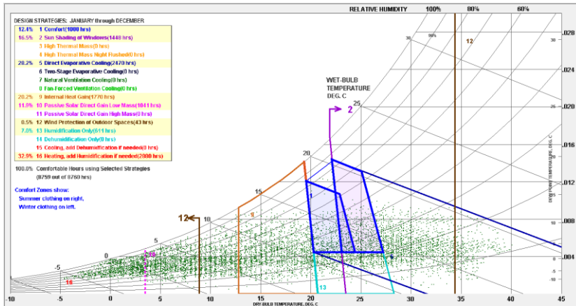
شکل ۹. نمودار سایکرومتریک شهر تهران (نگارندگان، از نرم‌افزار کلایمت کانسلانت)
