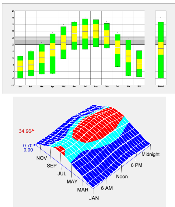
شکل ۱. میانگین دمای هوا؛ شکل ۲: چارت ۳ بعدی دمای هوای ماهانه
