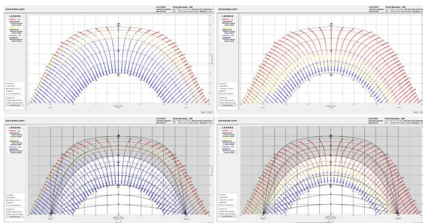
شکل ۵. بالا: دیاگرام خورشیدی؛ از چپ به راست: فصول گرم و سرد سال. پایین: تأثیر سایه‌بان؛ از چپ به راست: فصول گرم و سرد (نگارندگان، از نرم‌افزار کلاسیک کانسلانت)
