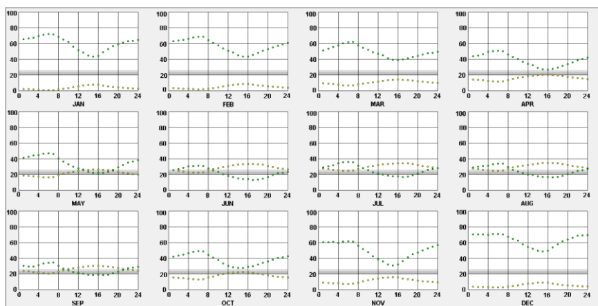
شکل ۶. مقایسه میزان رطوبت نسبی در ماه‌های مختلف سال (نگارندگان، از نرم‌افزار کلایمت کانسالنت)
