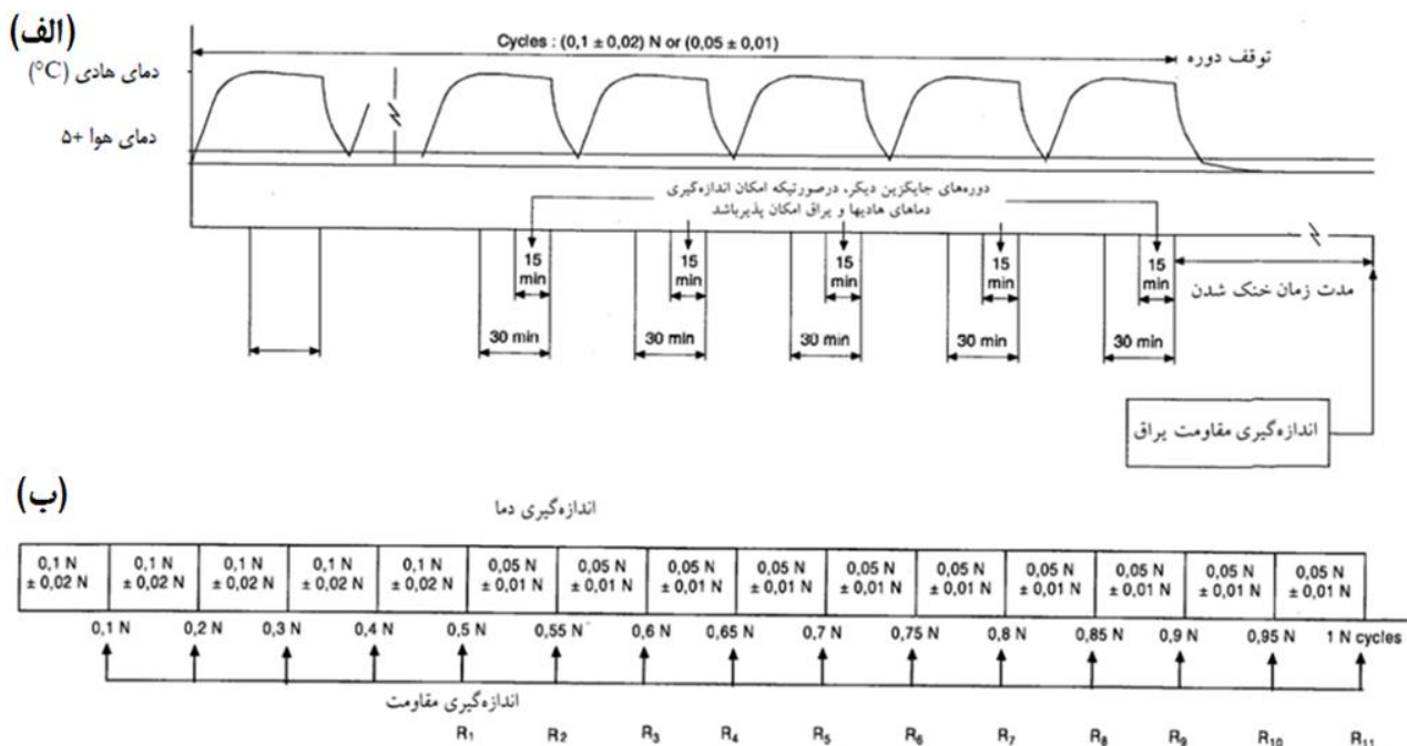
شکل ۴. (الف) سیکل‌های جریان/گرما اعمالی روی اتصالات در حین آزمون بیرسازی الکتریکی و (ب) بازه های زمانی اندازه گیری دما و مقاومت الکتریکی رابط ها و هادی های مرجع [۱۳]
