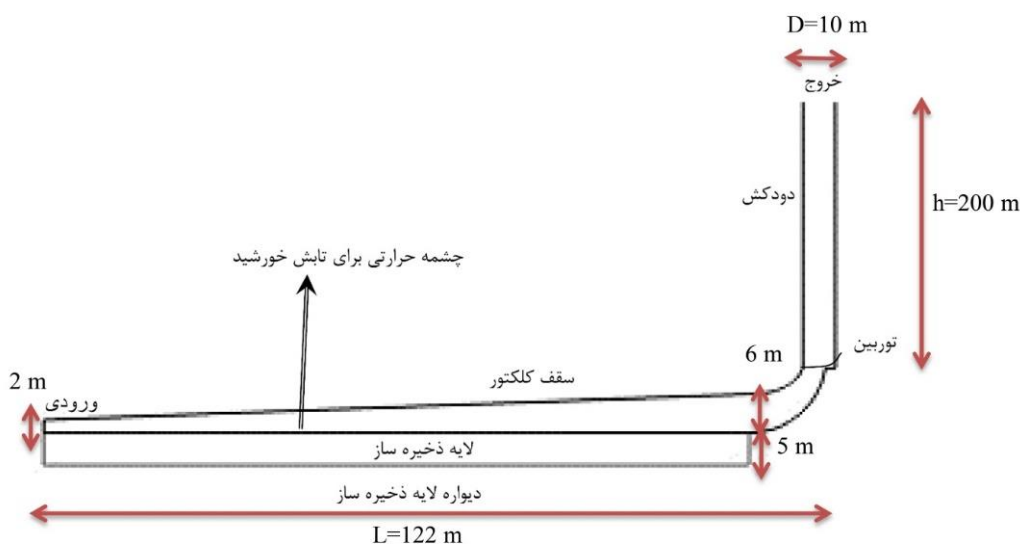
شکل ۲. مشخصات هندسی نیروگاه دودکش خورشیدی مورد مطالعه و مانرانا رس (اسپانیا)
