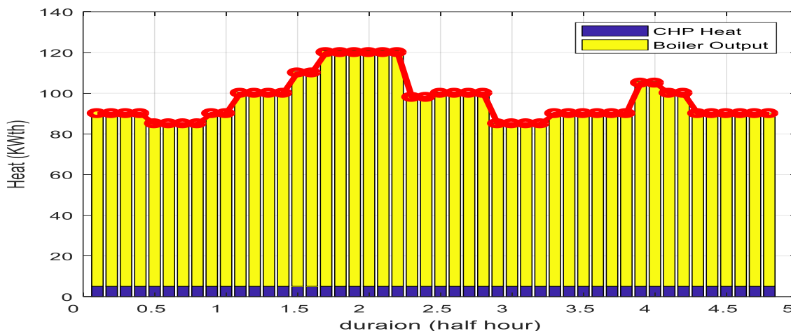
شکل ۱۲. توزیع گرمایشی سیستم مورد مطالعه در توان و ظرفیت CHP برابر ۱۰ کیلووات
