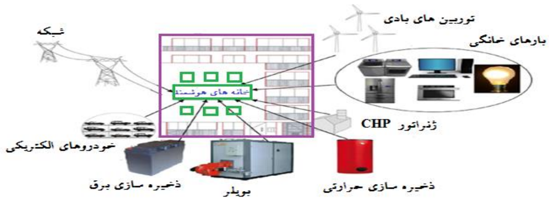
شکل ۹. سیستم مورد مطالعه (اویس ۹۰ و دیگران، ۲۰۱۸)
