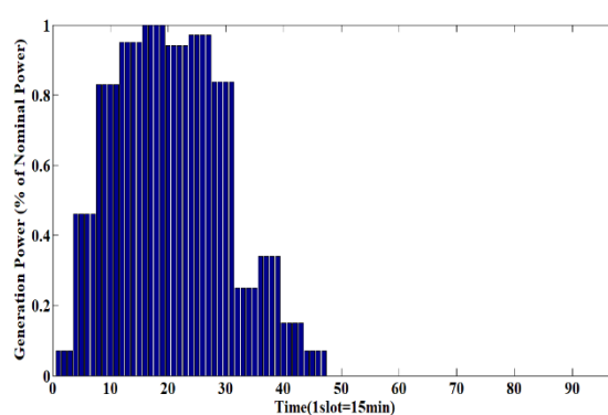
شکل ۷. رژیم تولید توان توربین بادی
