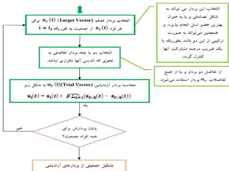
شکل ۳. فلوچارت عملگر جهش
