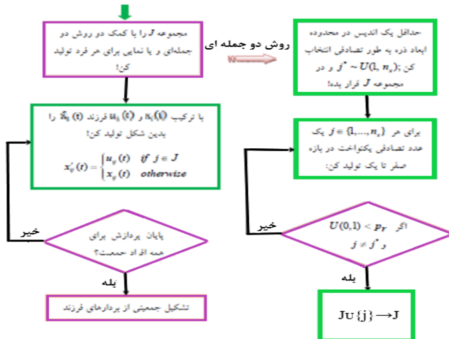
شکل ۴. فلوچارت برش دو جمله ای
