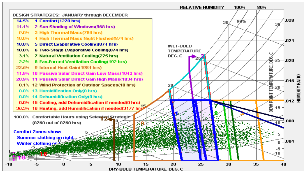
شکل ۹. چارت سایکرومتریک همدان (مرجع: نرم افزار کلایمت کانسالتنت)
