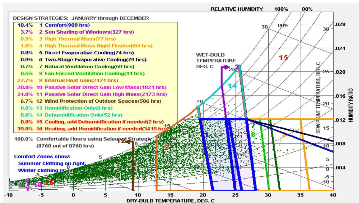
شکل ۹. ادامه شکل ۹. چارت سایکرومتریک اردبیل
