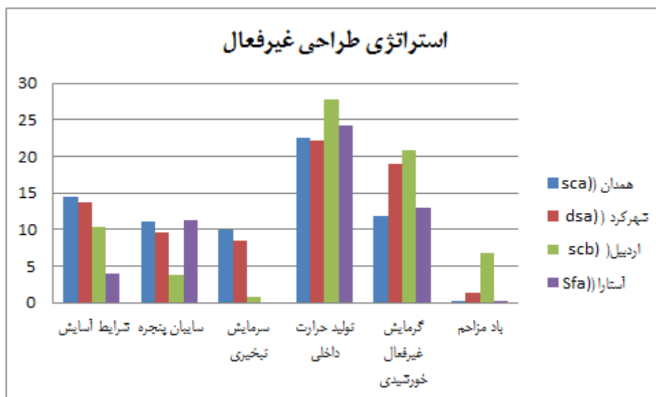
شکل ۱۱. استراتژی طراحی غیر فعال بر حسب درصد
