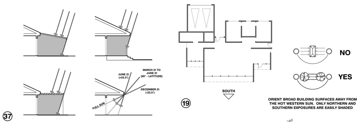
شکل ۱۲. تدبیر معماری الف) جهت قرارگیری پنجره ها ب) طراحی سایبان (مرجع: نرم افزار کلاسیت کانسلانت)
