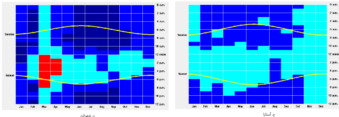
شکل ۵. میزان سرعت و درصد وزش باد (مرجع: نرم افزار کلایمت کانسالنت)
