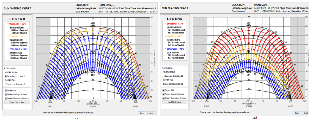
شکل ۷. الف) نمودار خورشیدی تابستان و پاییز (۲۱ ژوئن تا ۲۱ دسامبر) همدان ب) نمودار سایه خورشیدی زمستان و بهار (۲۱ دسامبر تا ۲۱ ژوئن) همدان
