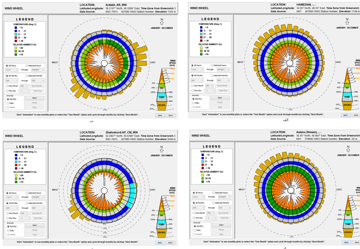
شکل ۸. چرخ باد الف. همدان ب. اردبیل ج. آستارا د. شهرکرد (مرجع: نرم افزار کلایمت کانسالنت)
