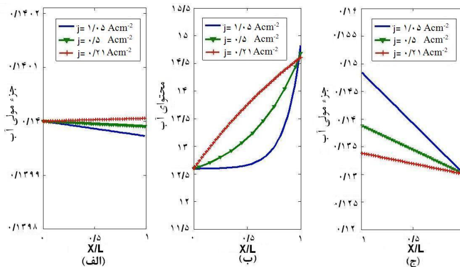
شکل ۱۳: توزیع آب در دانسیته جریان های 0.05 ، 0.5 و 2.1 \text{ Acm}^{-2}
