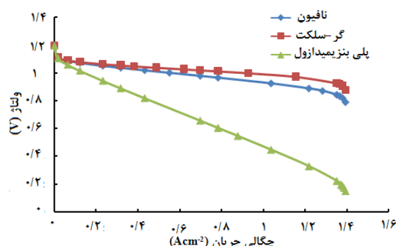
شکل ۷: منحنی قطبیدگی پیل سوختی برای سه غشاء پلیمری مختلف
