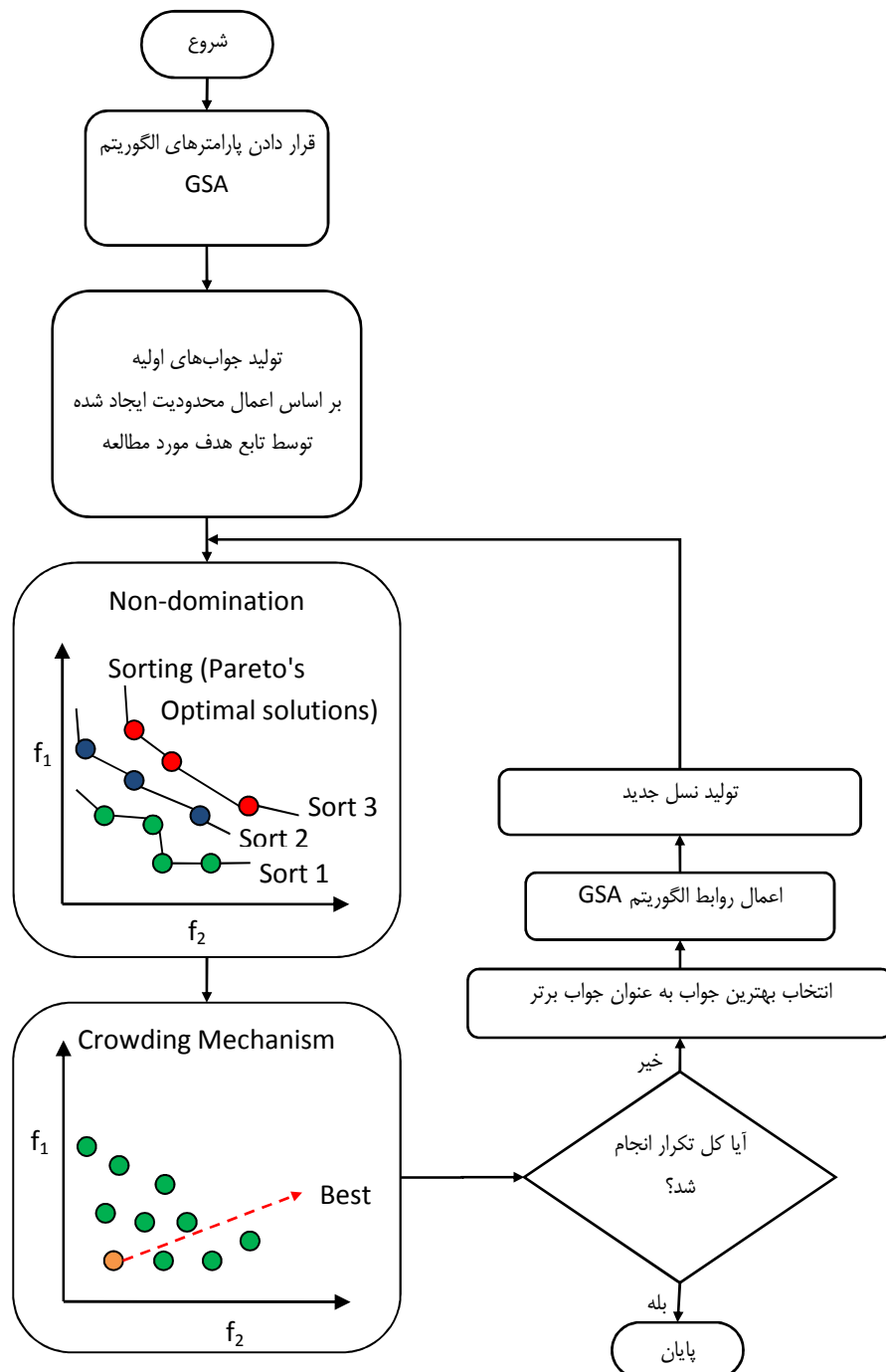
شکل ۲: فلوجارت الگوریتم پیشنهادی بر مساله EED
