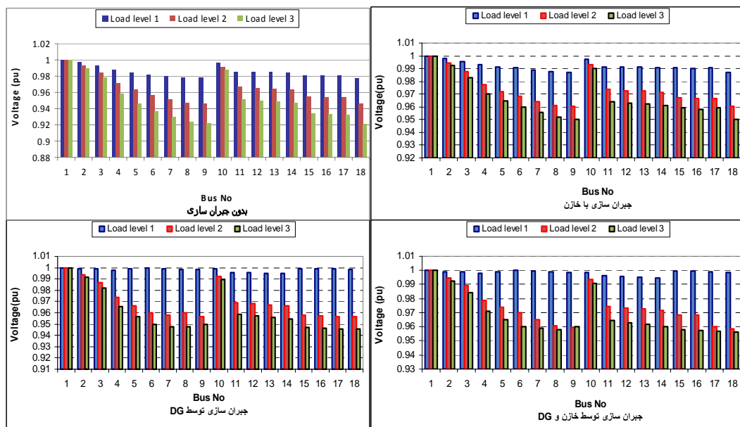
شکل ۱۲) پروفیل ولتاژ در چهار حالت عملکرد شبکه
