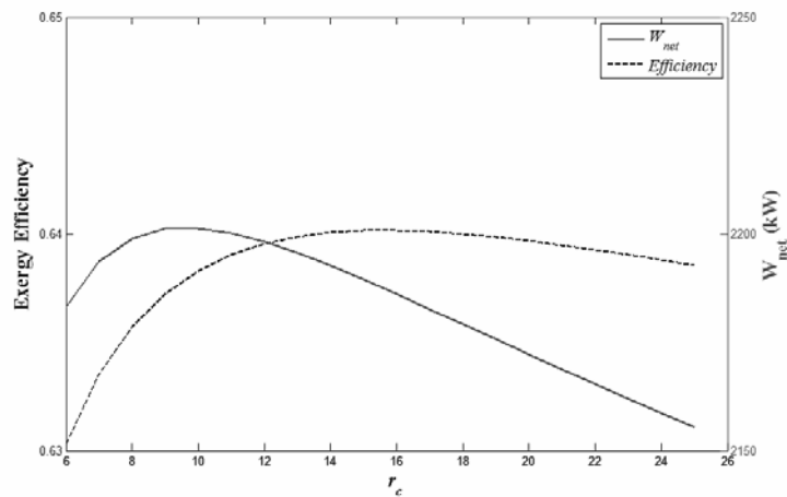
شکل ۵: تغییرات راندمان آگزردی و توان خالص خروجی با نسبت فشار کمپرسور
