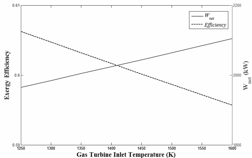
شکل ۶: تاثیر دمای ورودی به توربین گاز بر روی راندمان آگزردی و توان خالص خروجی
