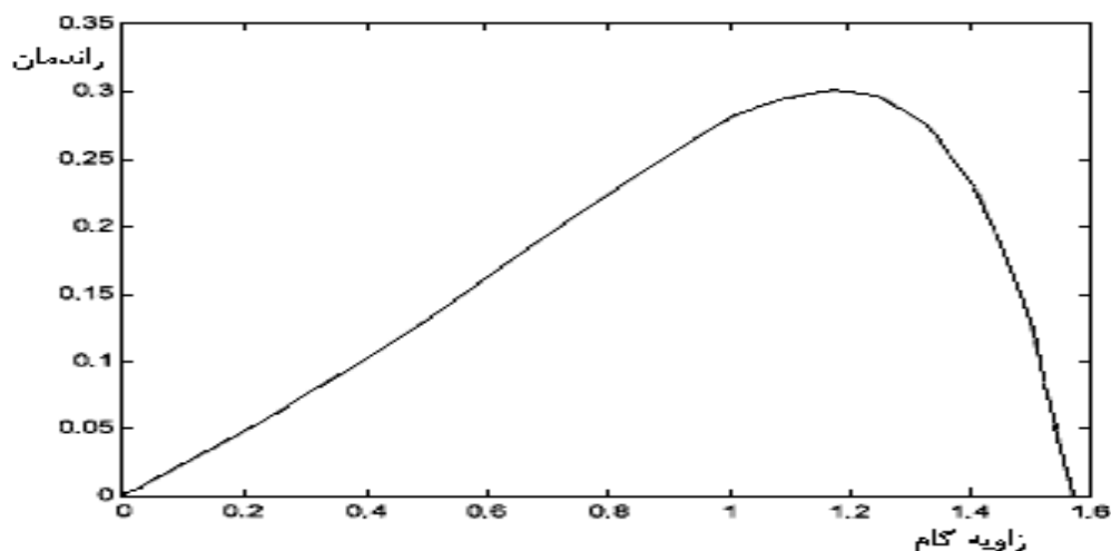
شکل ۷: راندمان \mathcal{E} بر حسب زاویه گام \varphi
