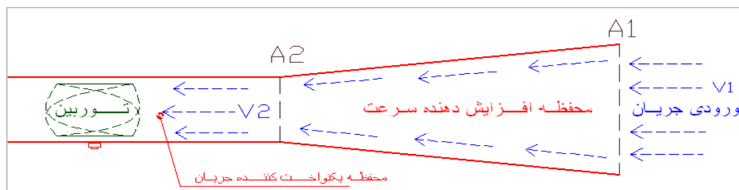
شکل ۱۱: حجم کنترل افزایش دهنده سرعت و محفظه یکنواخت کننده جریان موج جزر و مد
