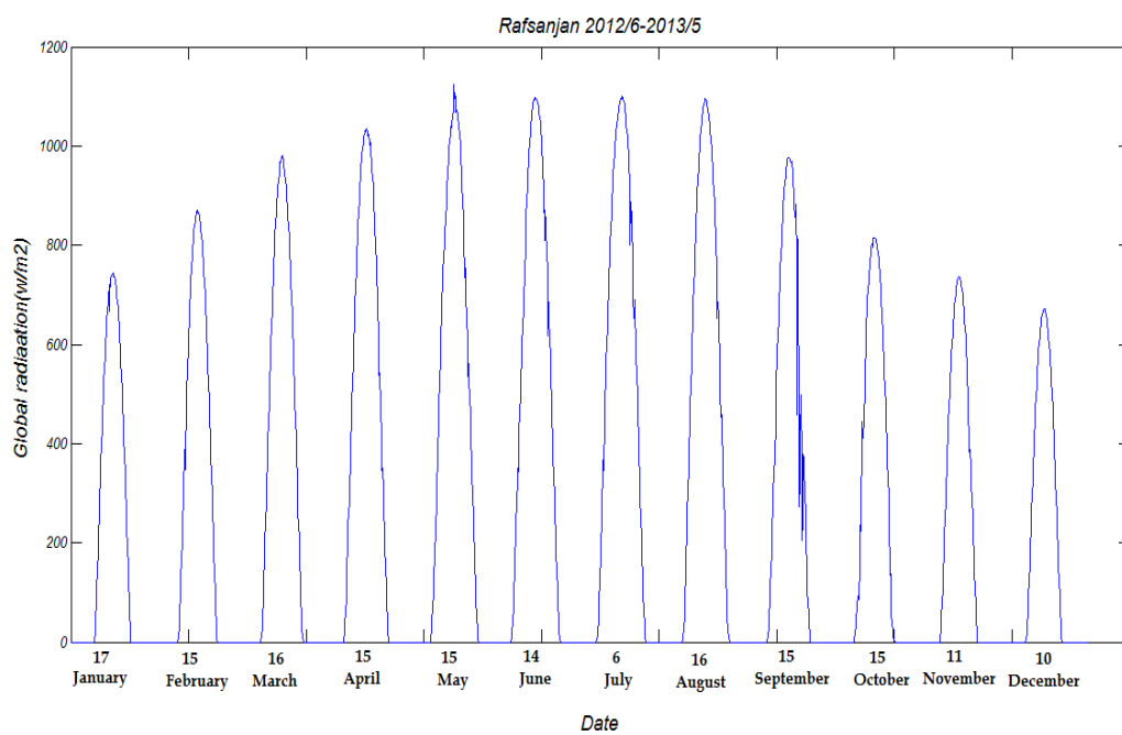
شکل ۴) تابش کل اندازه گیری شده توسط پیرانومتر ایستگاه سینوپتیک شهر رفسنجان برای یک روز از هر ماه
