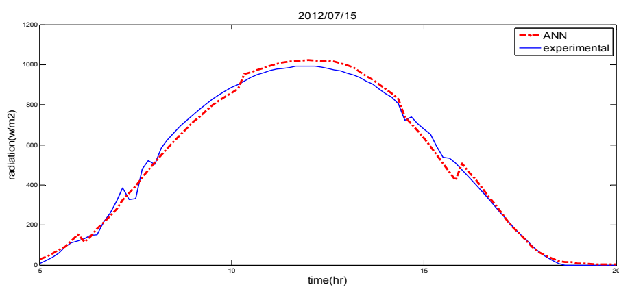
شکل ۱۵ مقایسه شبکه عصبی (ANN) با داده های اندازه گیری (experimental) شده برای یک روز از
