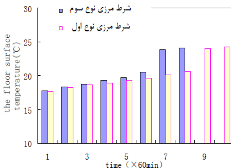
شکل ۳) رابطه دمای سطح کف و زمان ذخیره حرارت تحت شرایط مرزی مختلف
