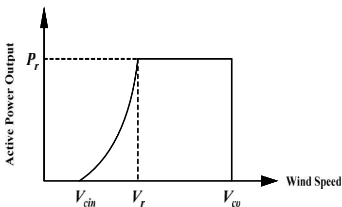
شکل (۱) مشخصه "توان-سرعت" توربین بادی
