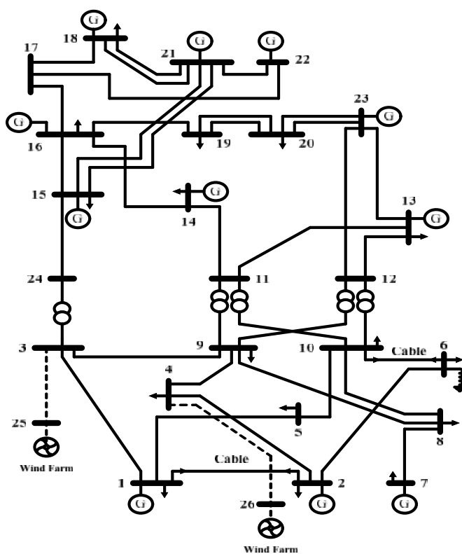
شکل ۵) شبکه ۲۴ باسه IEEE-RTS اصلاح شده
