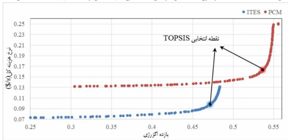
شکل (۴) منحنی بهینه سازی Pareto Front برای دو سیستم ITES و PCM
