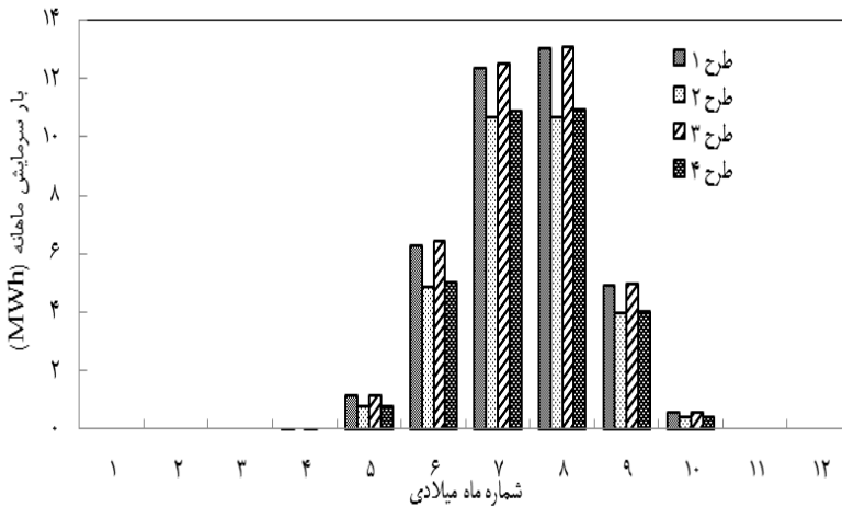
شکل ۱۰. بار سرمایه‌گذاری ماهانه در طرح‌های مختلف در تبریز
