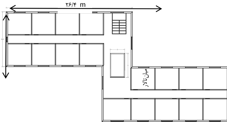
شکل ۱. پلان فضای نمونه مورد بررسی
