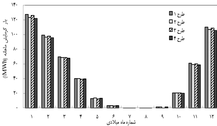
شکل ۹. بار گرمایش ماهانه در طرح‌های مختلف در تبریز
